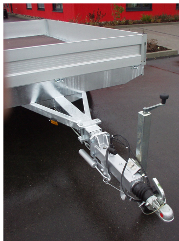
Stufenlos ausziehbare Deichsel Bremsgestänge stellt sich beim Verstellen der Deichsel mit ein
